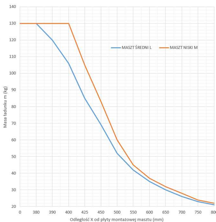
Wykres dopuszczalnego obciążenia
